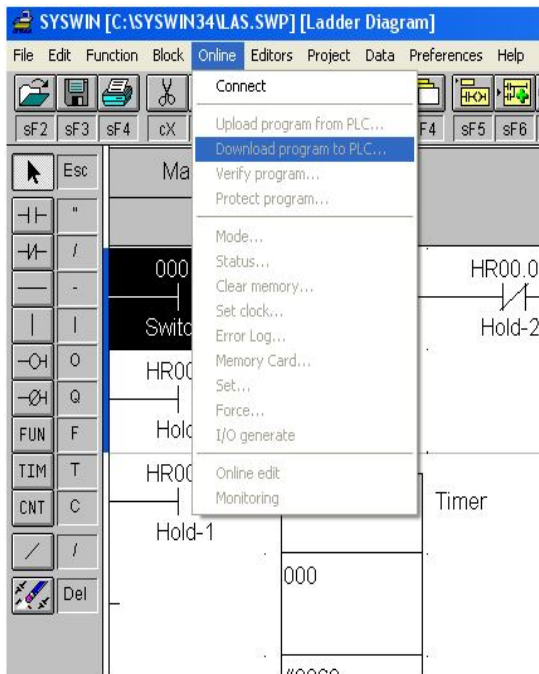
Gambar 4. Tampilan monitor untuk Down load program ke PLC
