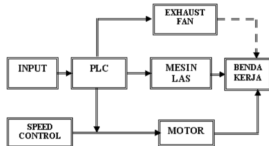
Gambar 2. Blok Diagram Pengelasan Secara Otomatis
