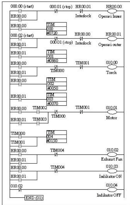
Gambar 3. Diagram Tangga
