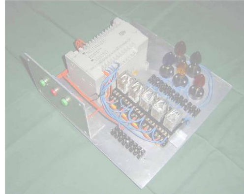
Gambar 5. Bentuk rangkaian kontrol yang dihasilkan dan dilengkapi dengan simulasi
