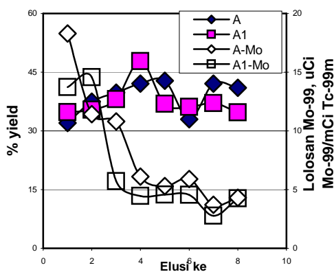
Gambar 2. Yield dan Lolosan ^{99}\text{Mo} dari sistem Generator ^{99}\text{Mo}/^{99\text{m}}\text{Tc} Berbasis PZC dengan pencucian menggunakan NaCl 0,9 % (A = yield generator A, A-Mo = lolosan ^{99}\text{Mo} pada generator A, A1 = yield generator A1, A1-Mo = lolosan ^{99}\text{Mo} pada generator A1)
