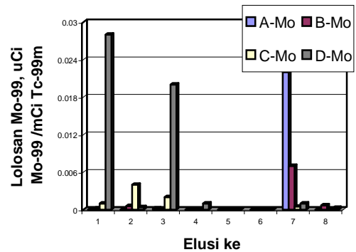
Gambar 6. Lolosan ^{99}\text{Mo} Pada Hasil Elusi ^{99}\text{Mo}/^{99\text{m}}\text{Tc} Dari Sistem Generator ^{99}\text{Mo}/^{99\text{m}}\text{Tc} Berbasis PzC (Poly Zirconium Compound) Dengan Kolom Alumina. (A-Mo Dan B-Mo = Lolosan ^{99}\text{Mo} Dari Kolom Dengan 1 G Alumina, C-Mo Dan D-Mo = Lolosan ^{99}\text{Mo} Dari Kolom Dengan 3 G Alumina)
