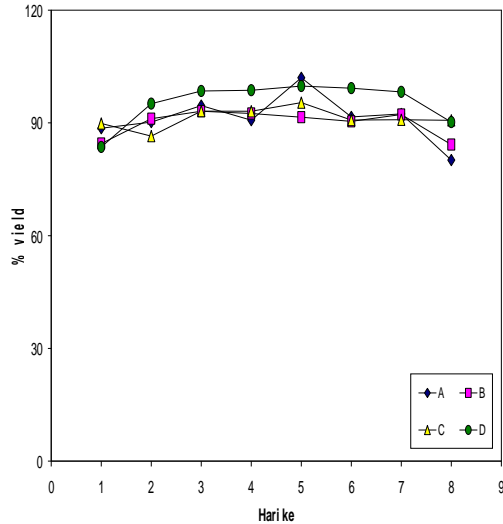
Gambar 5. Pengaruh pemakaian kolom alumina sebagai penangkap lolosan Mo-99 pada Generator ^{99}\text{Mo}/^{99\text{m}}\text{Tc} berbasis PZC (A dan B = kolom dengan berat alumina 3 g, C dan D = kolom dengan berat alumina 1 g)
