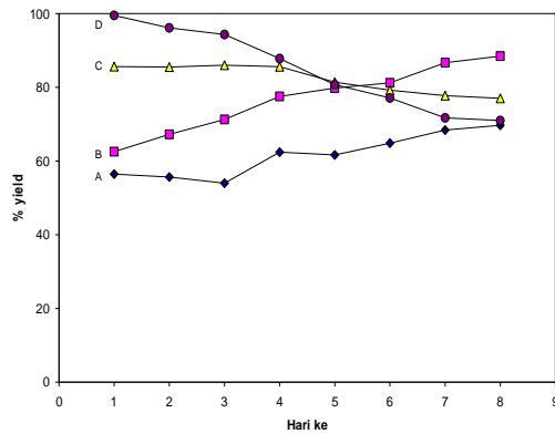
Gambar 3. Pengaruh pencucian dengan variasi kadar NaOCl terhadap yield molibdenum pada Generator ^{99}\text{Mo}/^{99\text{m}}\text{Tc} berbasis PZC (A = dengan NaOCl 0,05 % , B = dengan NaOCl 0,1 % , C = dengan NaOCl 0,5 % ) , D = dengan NaOCl 1 %)
