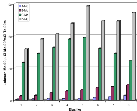
Gambar 4. Pengaruh pencucian dengan variasi kadar NaOCl terhadap lolosan Mo-99 ( Mo-99 breakthrough ) pada sistem Generator ^{99}\text{Mo}/^{99\text{m}}\text{Tc} berbasis PZC (A = dengan NaOCl 0,05 % , B = dengan NaOCl 0,1 % , C = dengan NaOCl 0,5 % ) , D = dengan NaOCl 1 %)
